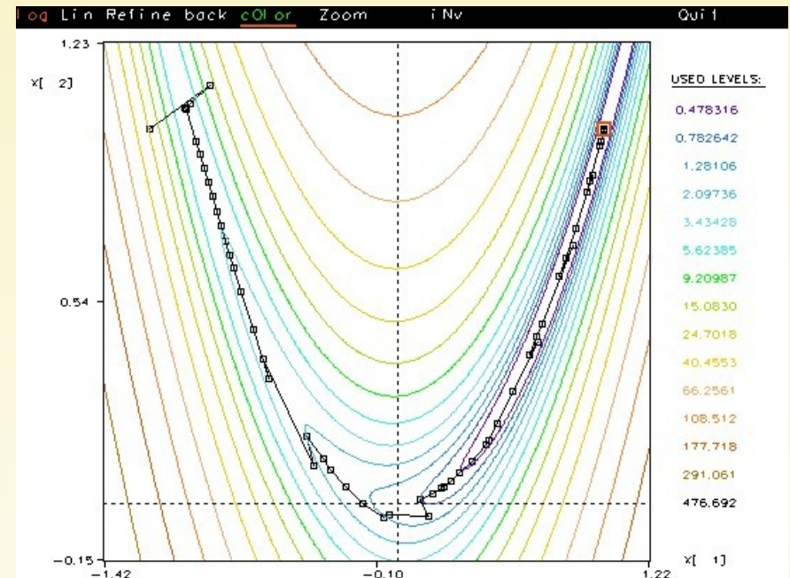
Rosenbrockova funkce
